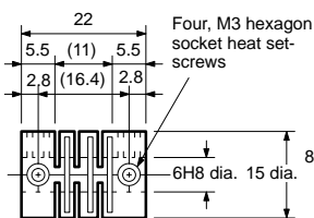
E69-C06B
