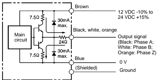
E6C2-CWZ5GH
